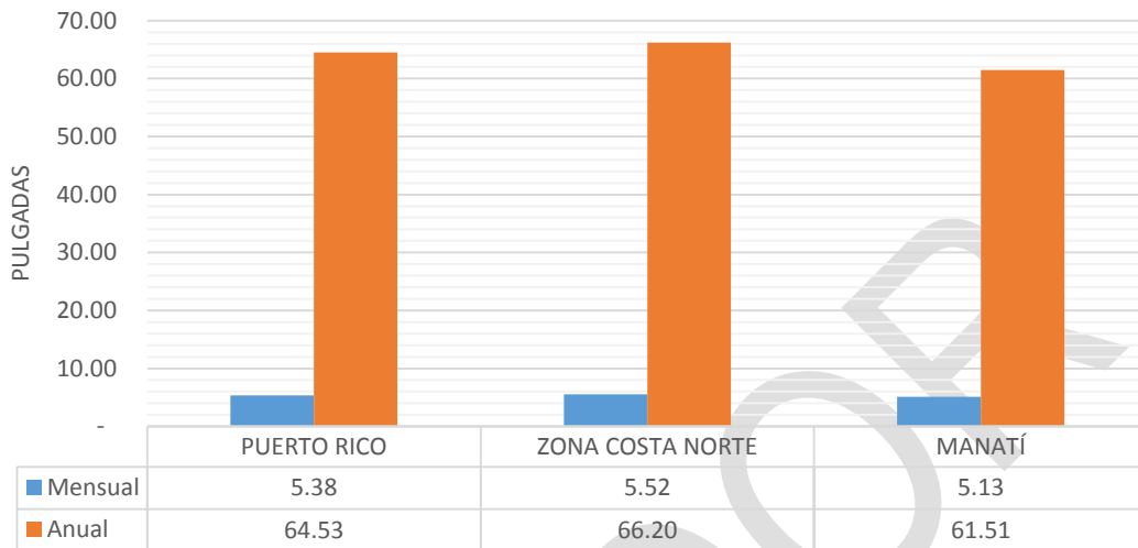
Gráfica 1. Precipitación promedio normal
